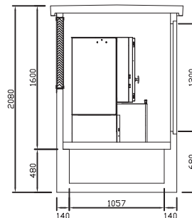
SECCION LATERAL
