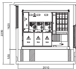
SECCION LONGITUDINAL
