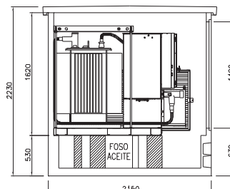
SECCION LATERAL
